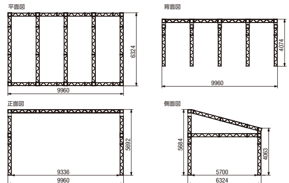
■3K×5K 外形図
