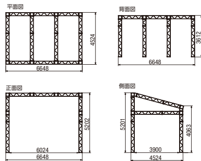
■2K×3K 外形図
